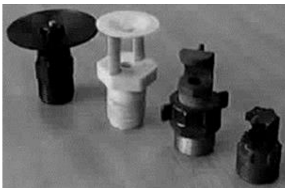
Рисунок 1 – Дефлекторные насадки (две слева – кругового и две справа – секторного действия)
