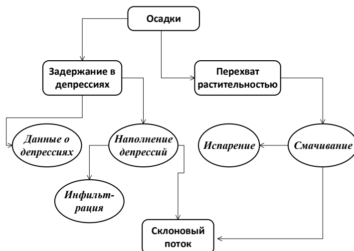
Рисунок 1 – Орграф начальной стадии формирования стока
